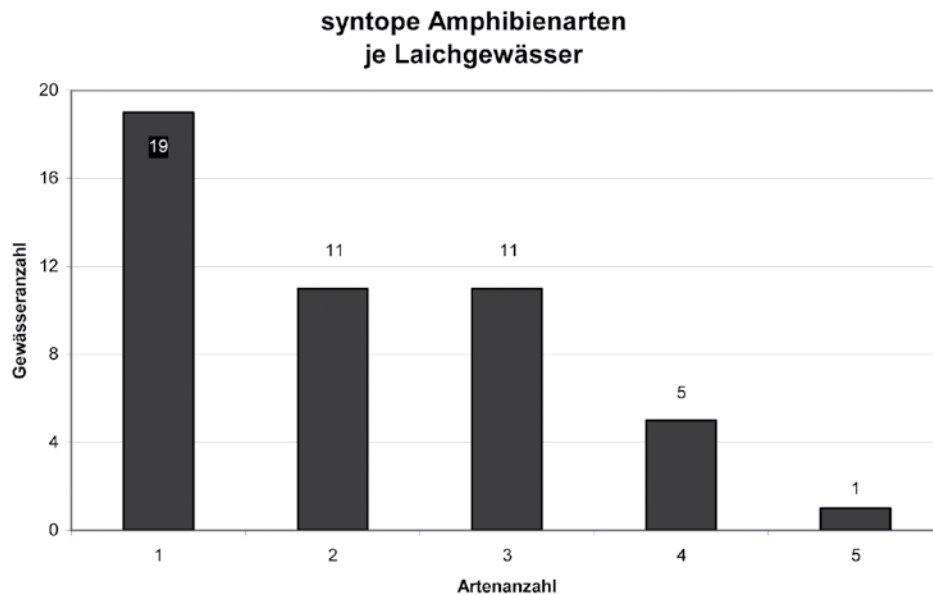
Abb. 6: Aufteilung der Anzahl von syntopen Amphibienarten in Laichgewässern des Springfrosches
