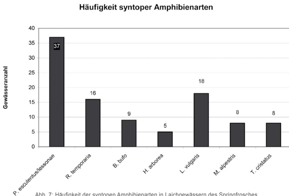
Abb. 7: Häufigkeit der syntopen Amphibienarten in Laichgewässern des Springfrosches
