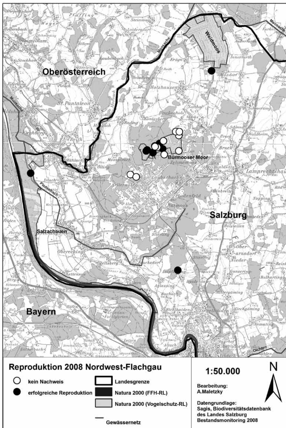
Abb. 9: Reproduktionserfolg des Springfrosches im Northwest-Flachgau 2008
